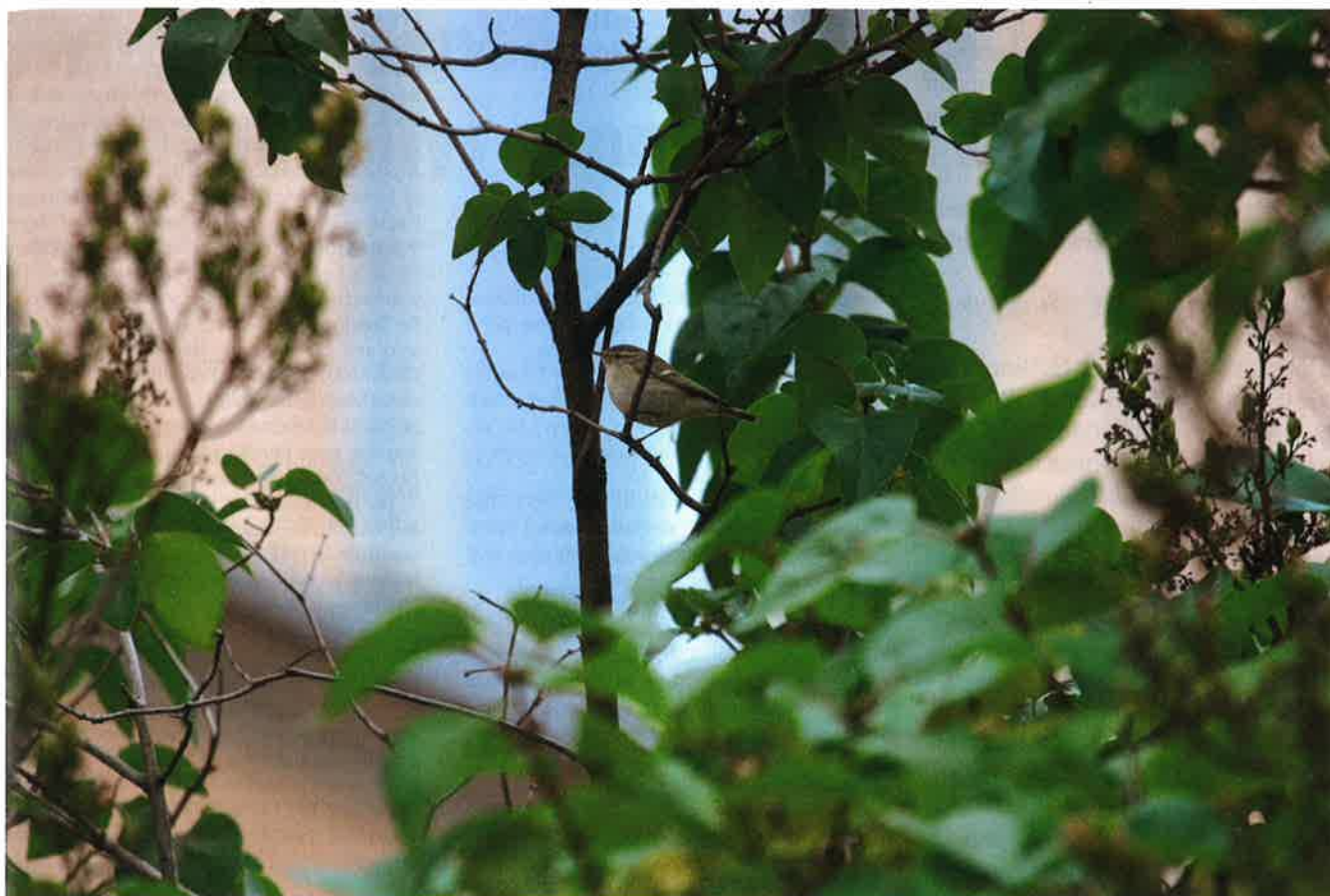
Kashmirinuunilintu ( Phylloscopus humei ) Helsingissä 18.10.2003. Lehvästössä vilkkaasti liikkuvaa "pienää vihreää" on vaikea seurata, joten hyvän kirjallisen kuvauksen laatiminen voi olla hankalaa. Kutsuäänten tuntemus helpottaa kuitenkin määrittystä. © Sampo Laukkanen — Hume's Leaf Warbler
