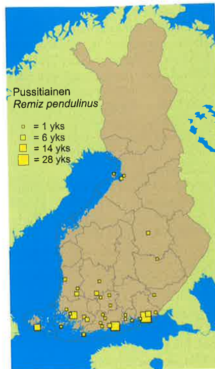
Viitatieäisen ( Parus palustris ) ja pussitieäisen ( Remiz pendulinus ) esiintyminen Suomessa. – Marsh Tit (left) and Penduline Tit (right) in Finland.
